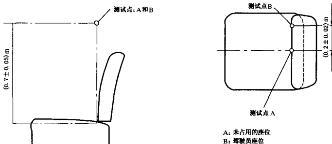
图 1 传声器相对于座椅的位置
